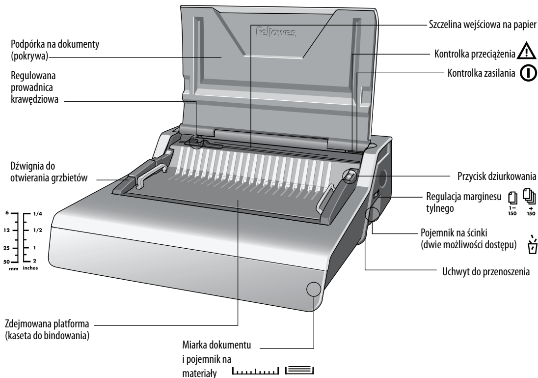
Pojemnik na grzbiecy i miarka dokumentu
