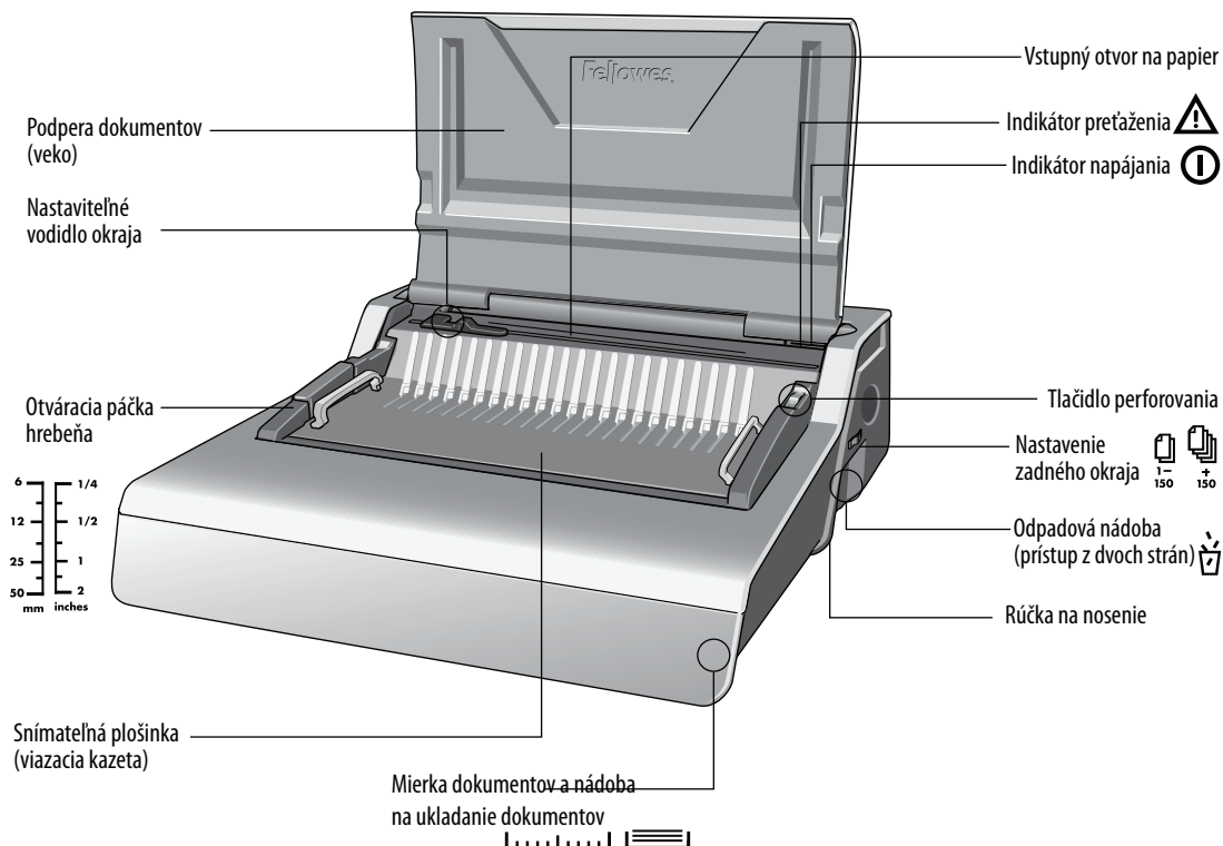
Snímateľná plošinka (viazacia kazeta)
