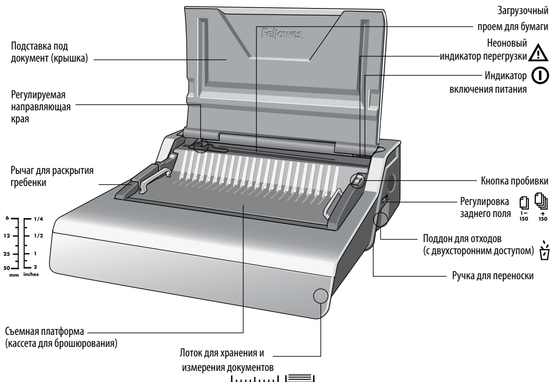
Съемная платформа (кассета для брошюрования)
