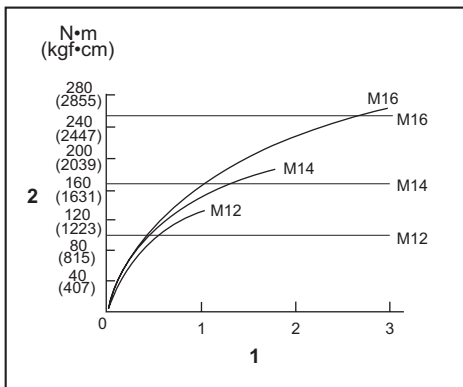
1. Anzugszeit (Sekunden) 2. Anzugsmoment
